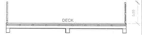
3 FACHADA FRENTE 1 : 50
